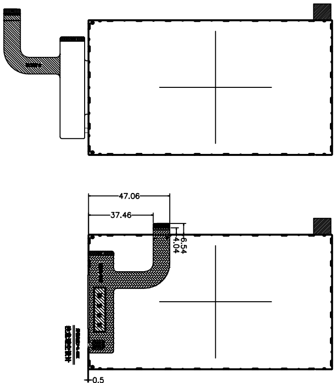
弯折示意图 弯折出货
